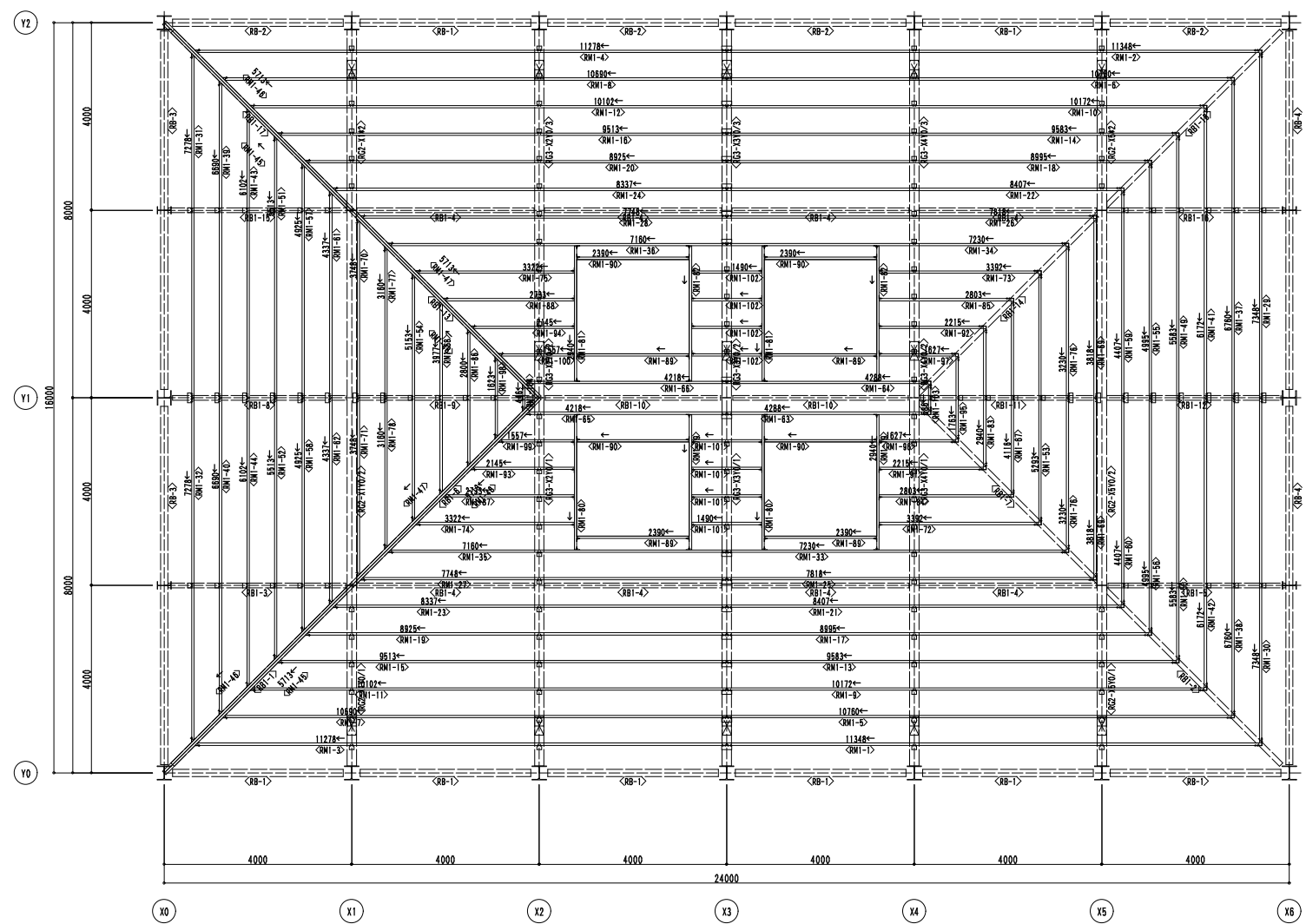
R 階 母屋割付図
