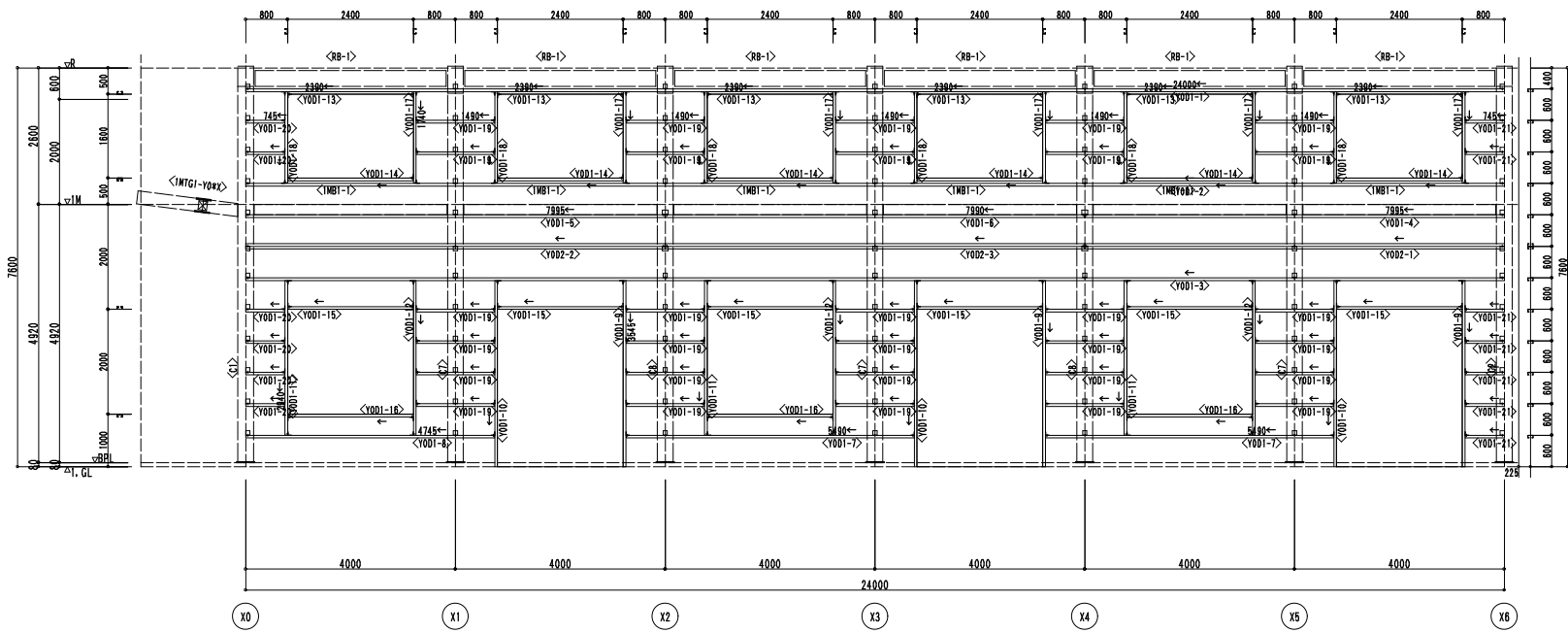
Y0 通り 胴縁割付図 1 胴縁 (D1) C - 100x 50x 20x 4.5 (D2) T I - 100x 50x 20x 4.5
