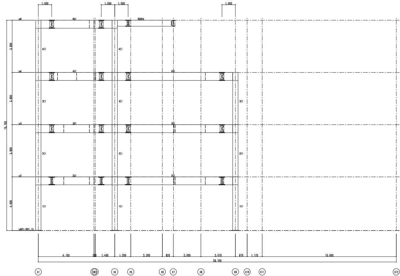
Y4 连廊 结构图
